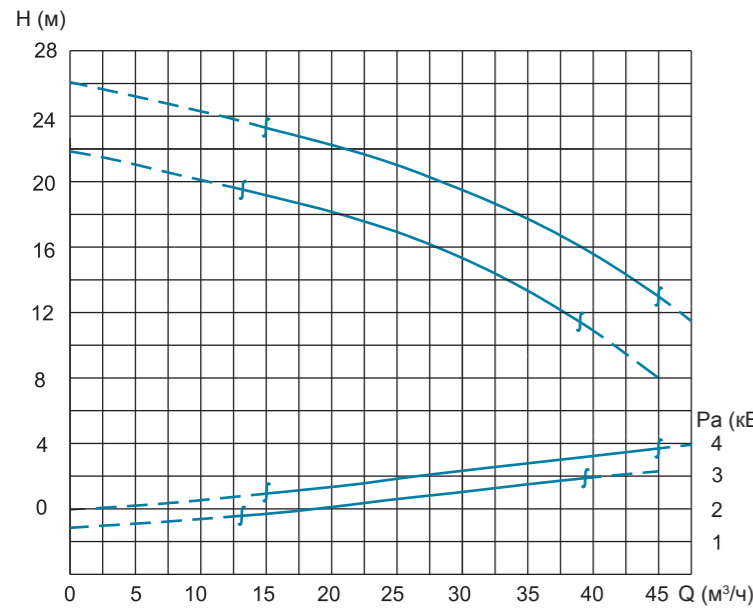
Кривая производительности
